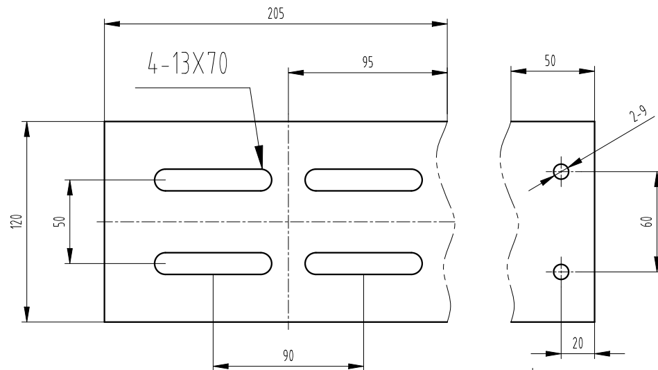
安装板件1 每台1件
