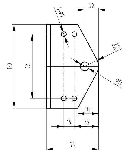
安装板件2 每台1件
