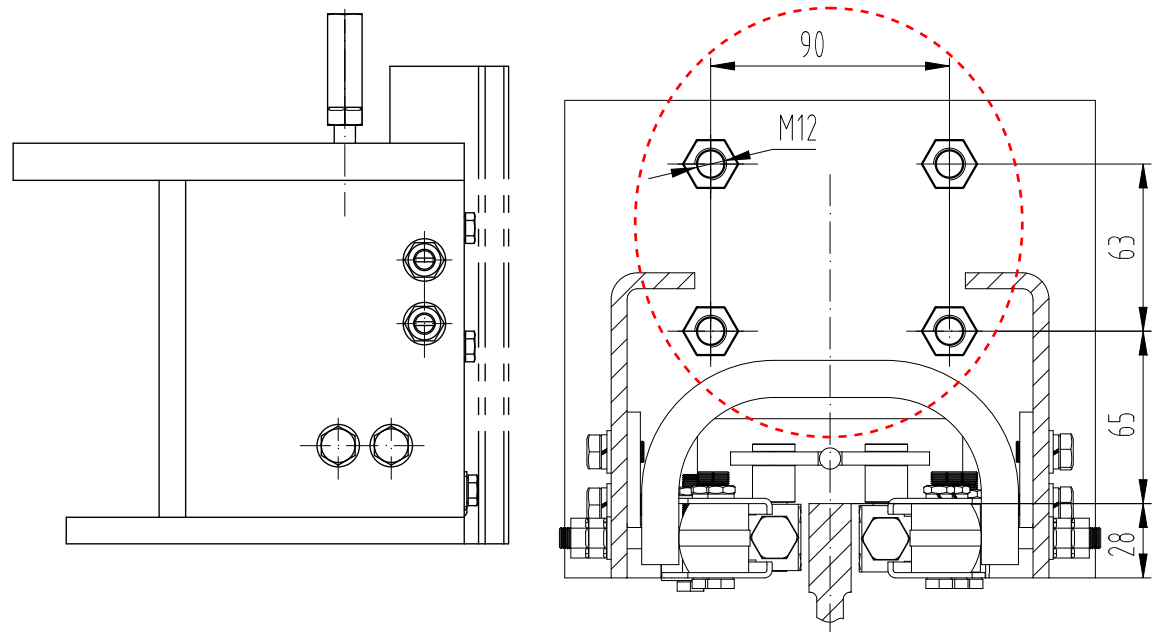
A向视图
