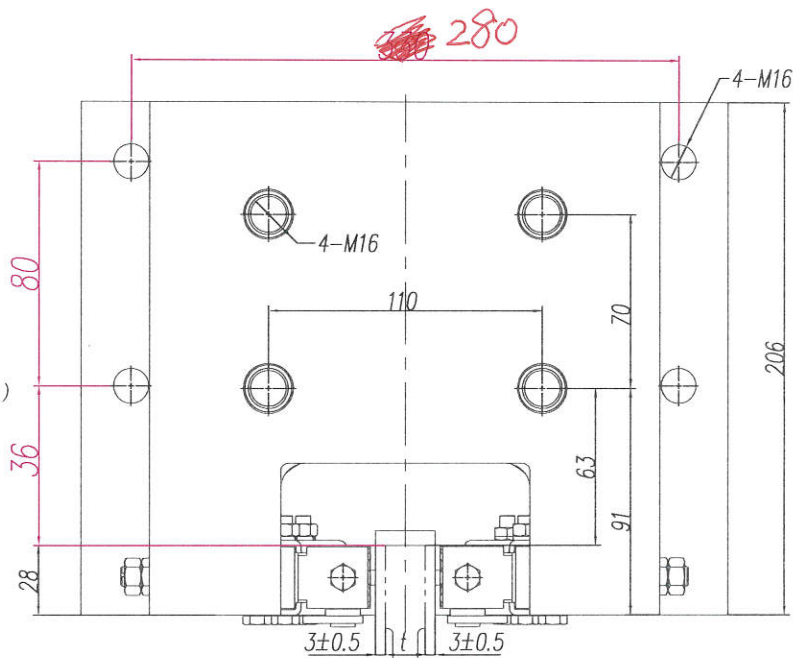
A 视图
