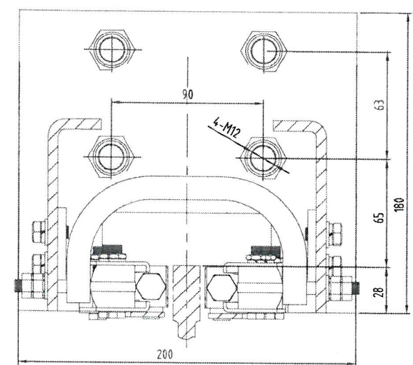
剖面 A-A
