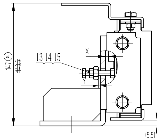
尺寸
