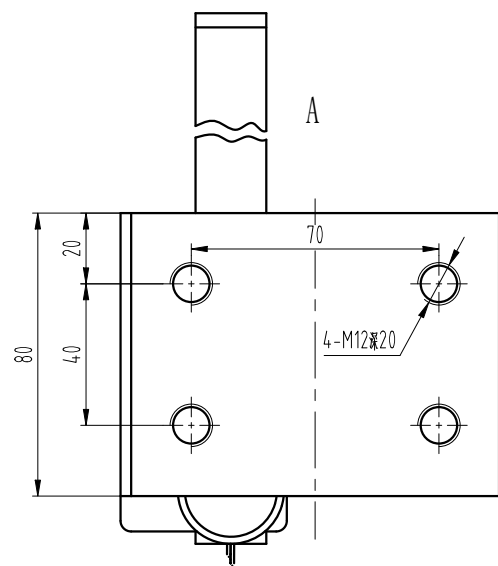
尺寸表
