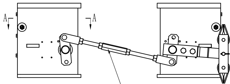
左右旋螺母 (花篮螺栓)
