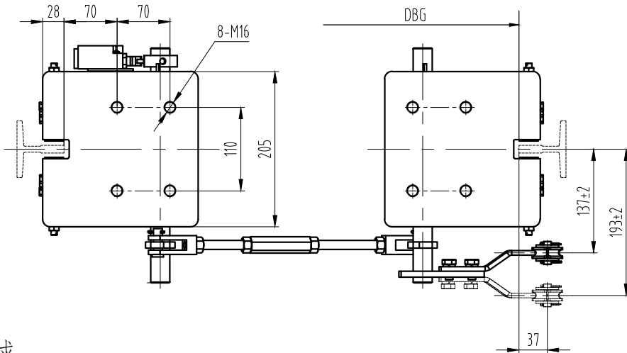
左右旋螺母 (花篮螺栓)
