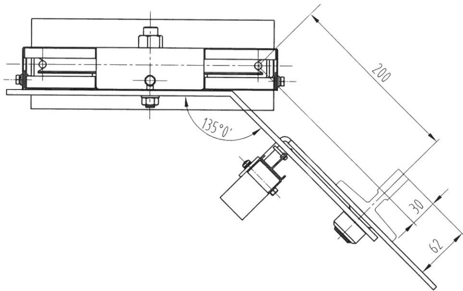
OX-300(45ZC)涨紧轮 铸铁30KG, 240-8, AD=200,DX=30
