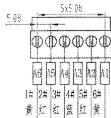
接插件接线示意图
