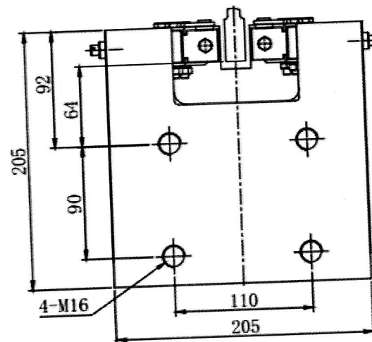
A向视图
