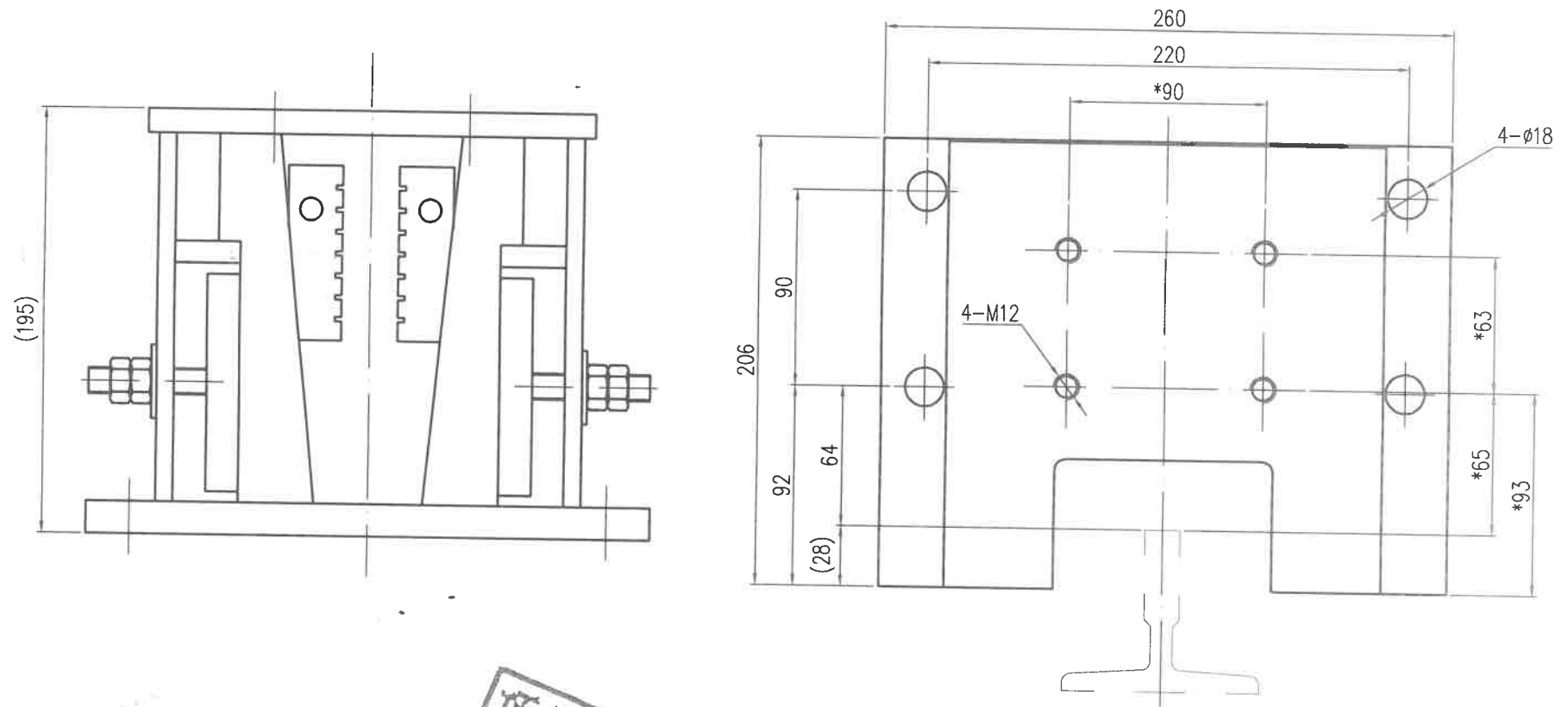
连接孔位示意图
