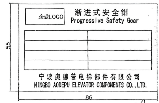
铭牌示意图
