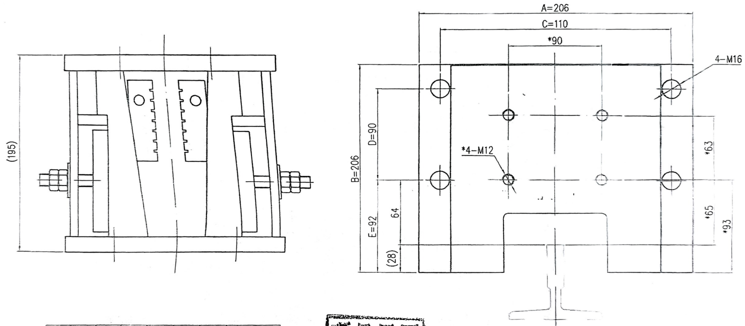
连接孔位示意图
