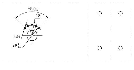
开孔尺寸
