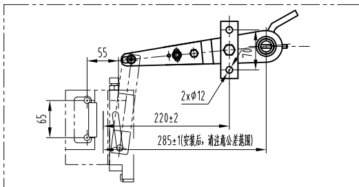
开孔尺寸
