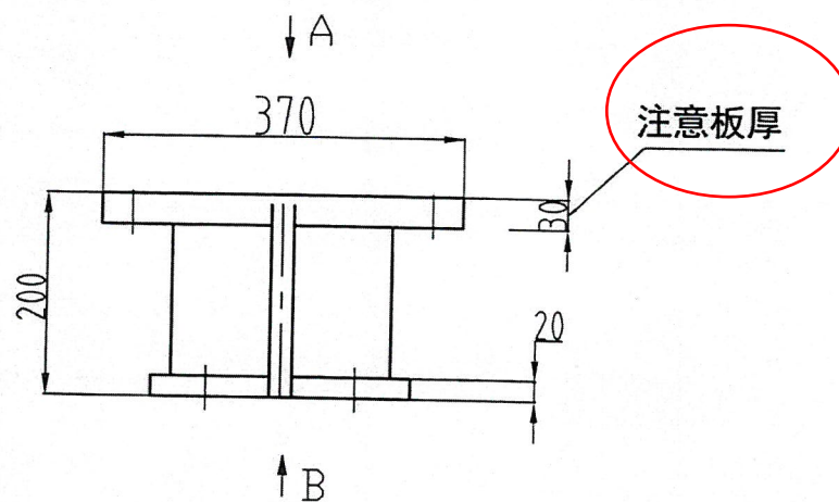
B向导靴连接
