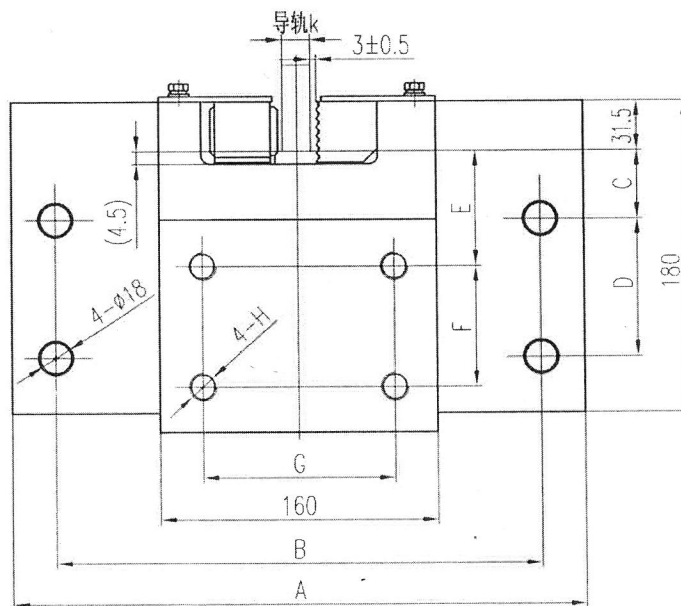
A向视图
