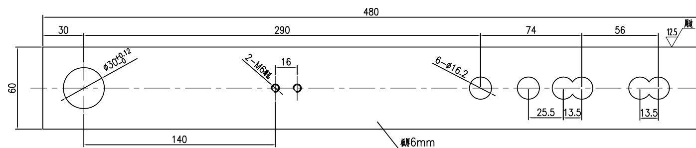
摇杆板件 奥德普型号: 0X-300D-2
