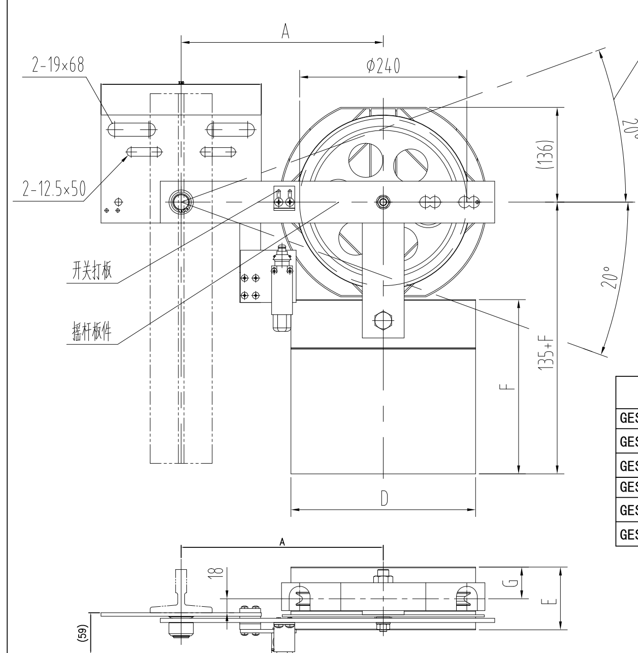
摇杆板件 奥德普型号: 0X-300D-2
