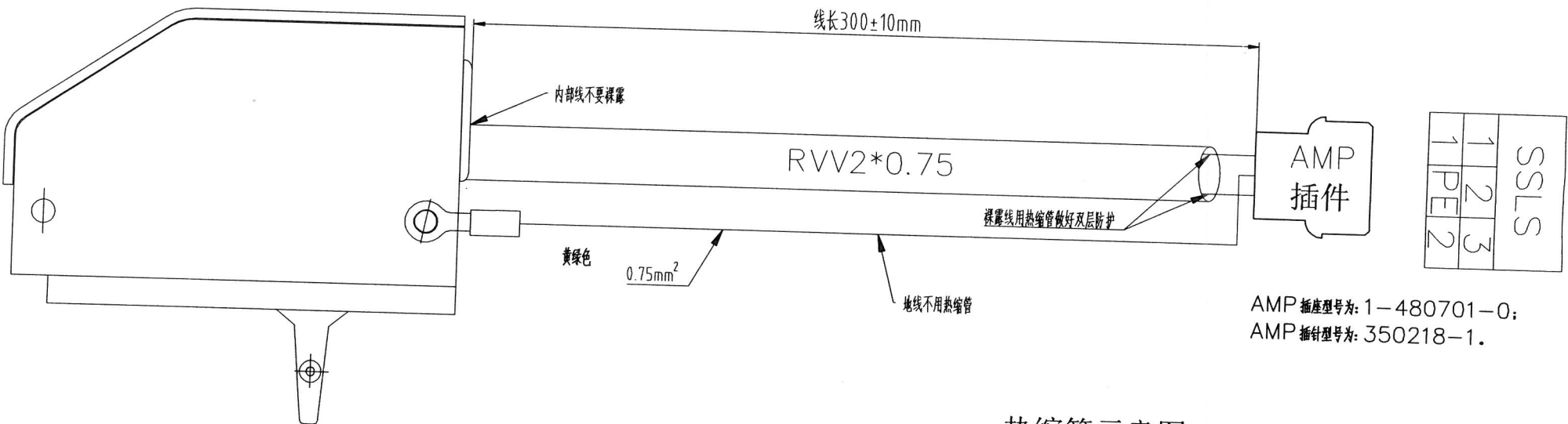
热缩管示意图
