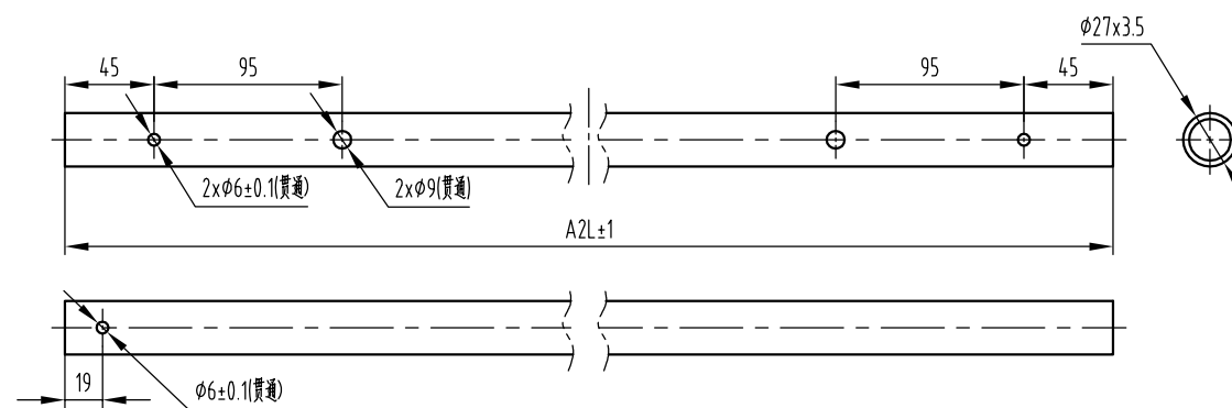
连接圆管开孔图
