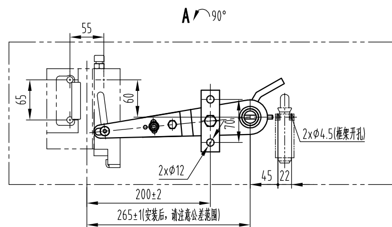
开孔尺寸
