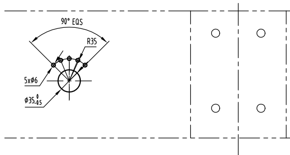
开孔尺寸
