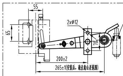
开孔尺寸
