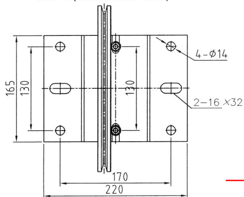
视图 A(去限速器主体配件)
