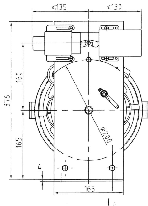
视图 A(去限速器主体配件)
