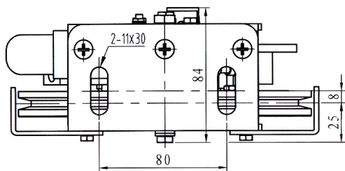
A向 (底板安装尺寸)
