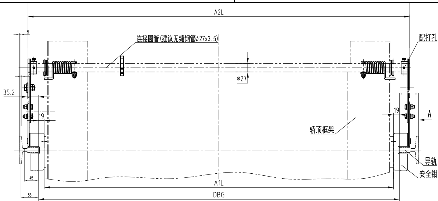
连接圆管开孔图
