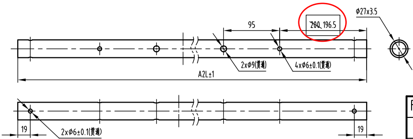
连接圆管开孔图
