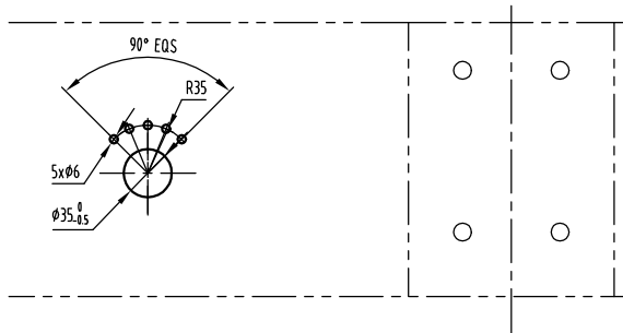
开孔尺寸
