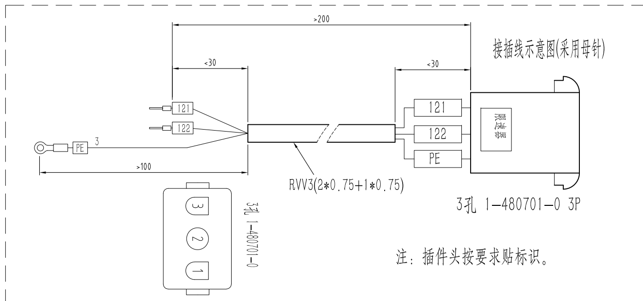
接插件示意图
