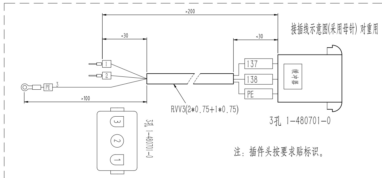
接插件示意图
