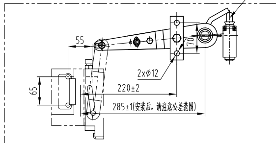
开孔尺寸
