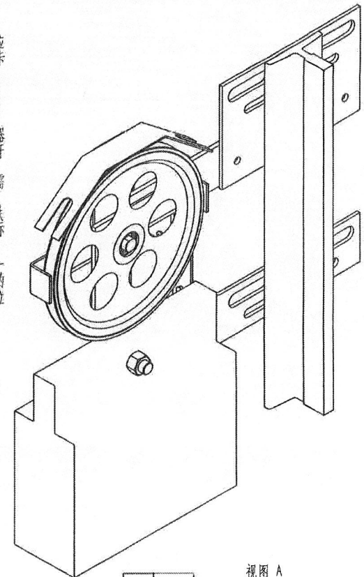
视图 A
