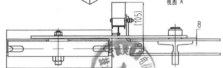
视图 A
