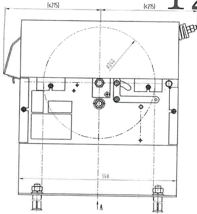
A(安装孔)
