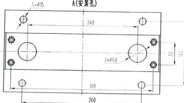
A(安装孔)
