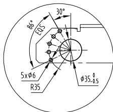
开孔尺寸
