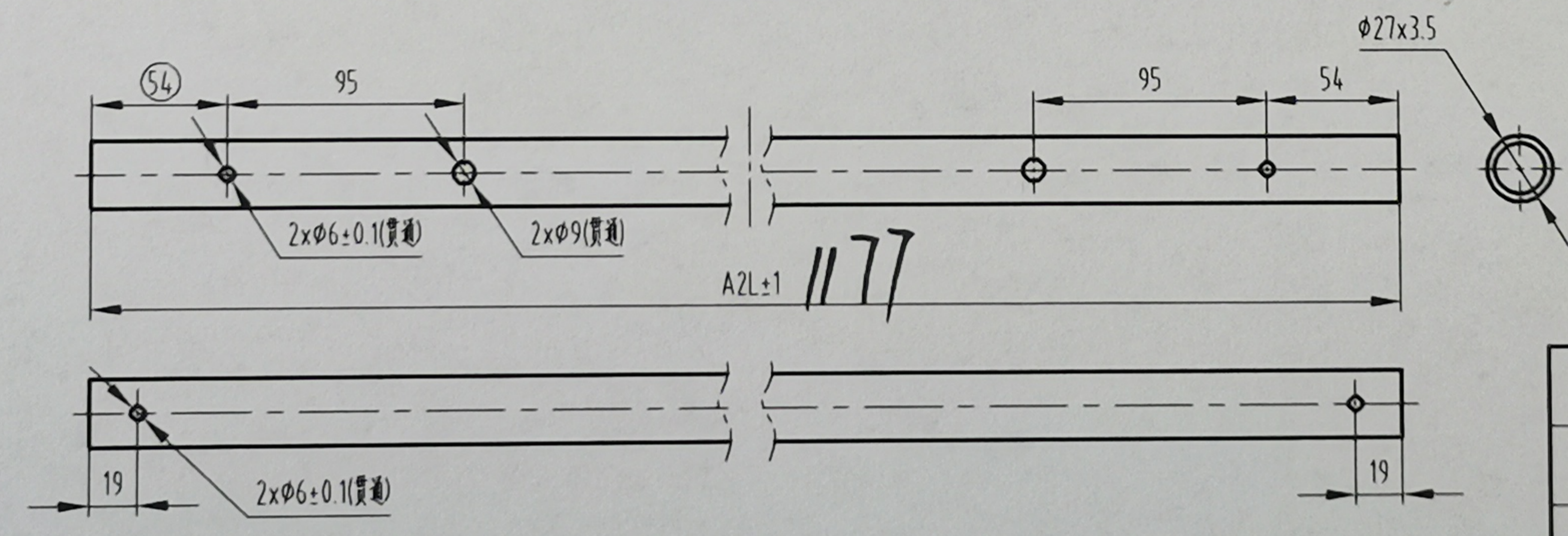
连接圆管开孔图
