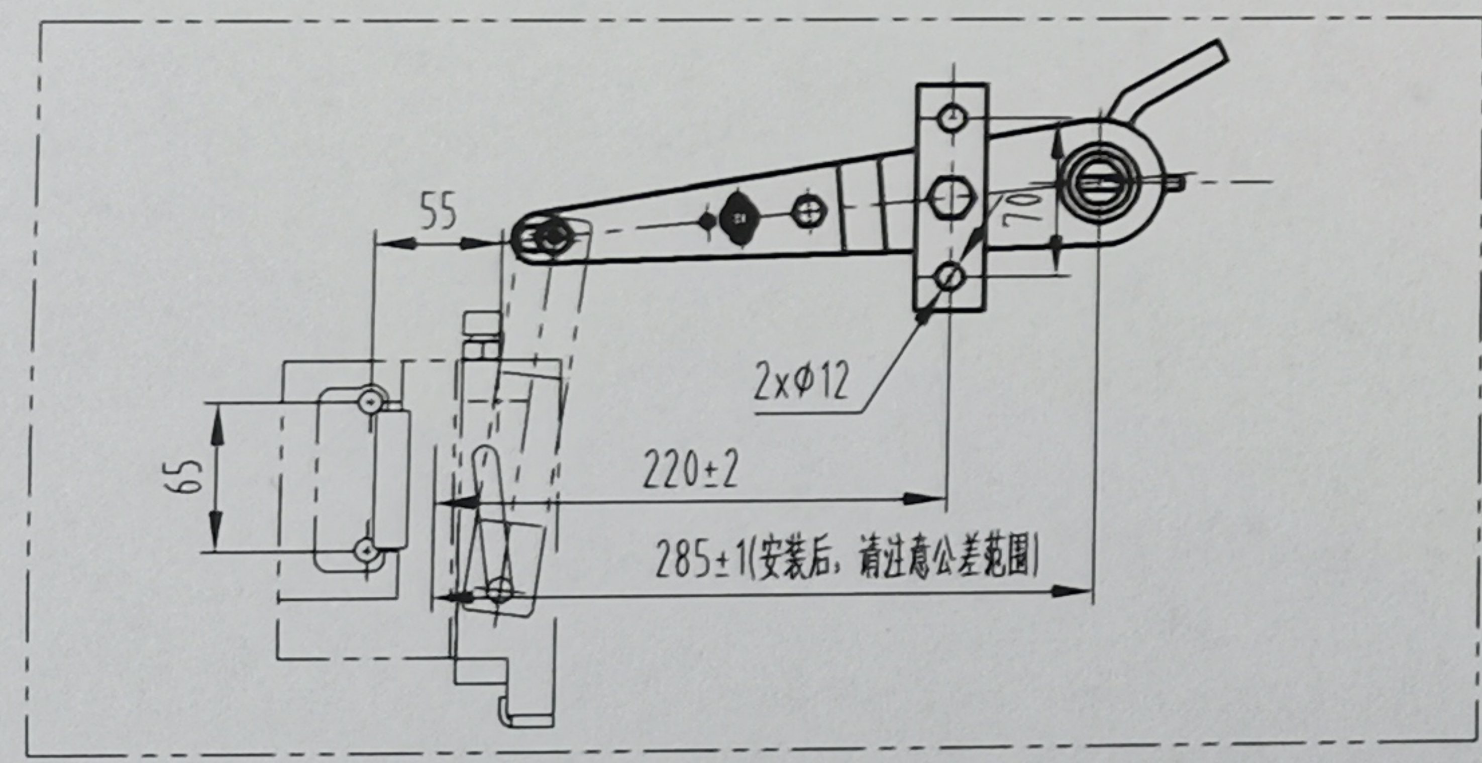
开孔尺寸
