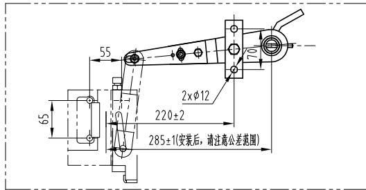
开孔尺寸
