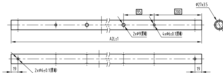
连接圆管开孔图
