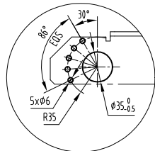
开孔尺寸
