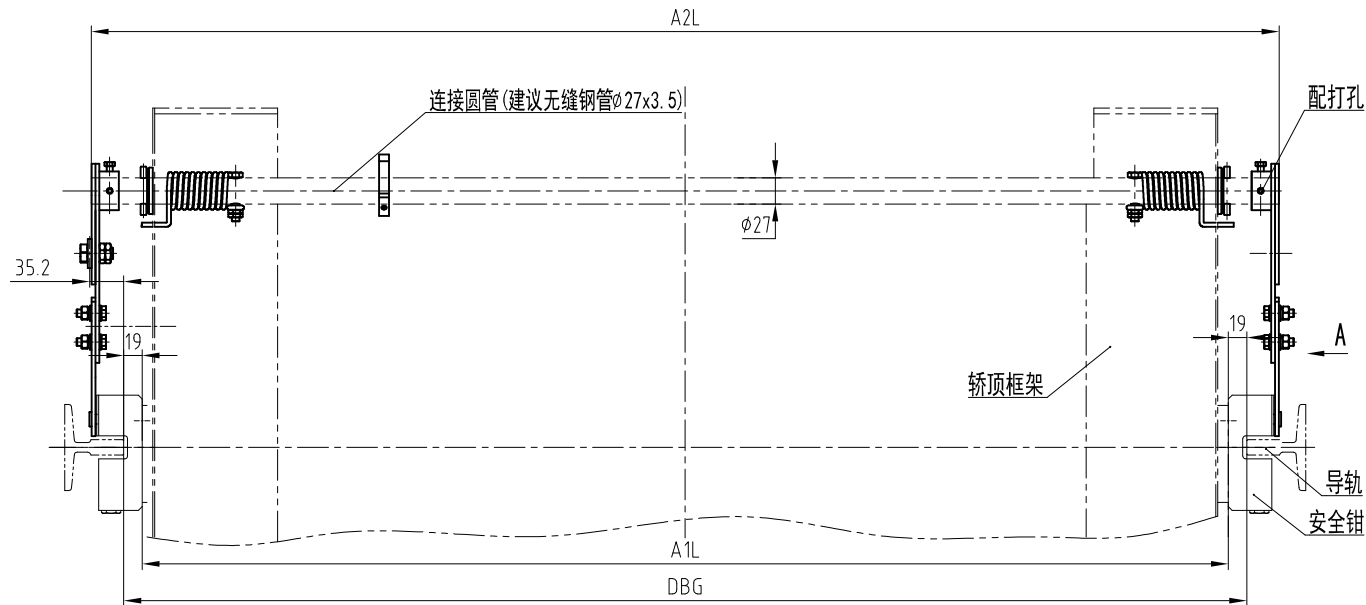
连接圆管开孔图
