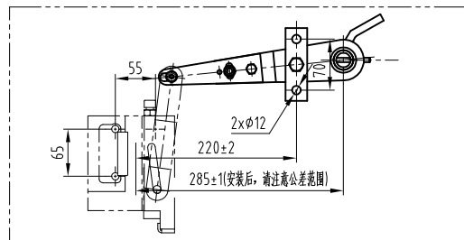
开孔尺寸
