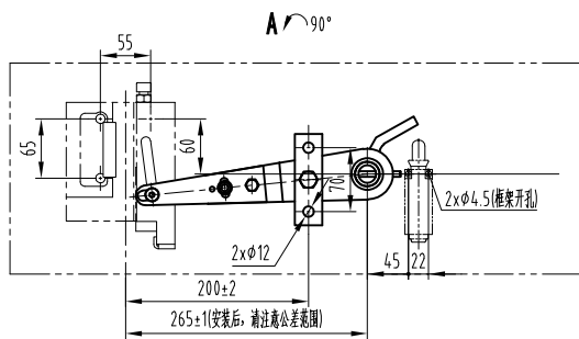
开孔尺寸
