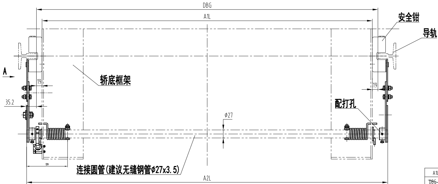
连接圆管开孔图
