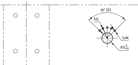
开孔尺寸
