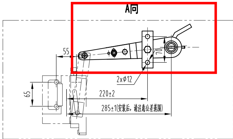
开孔尺寸
