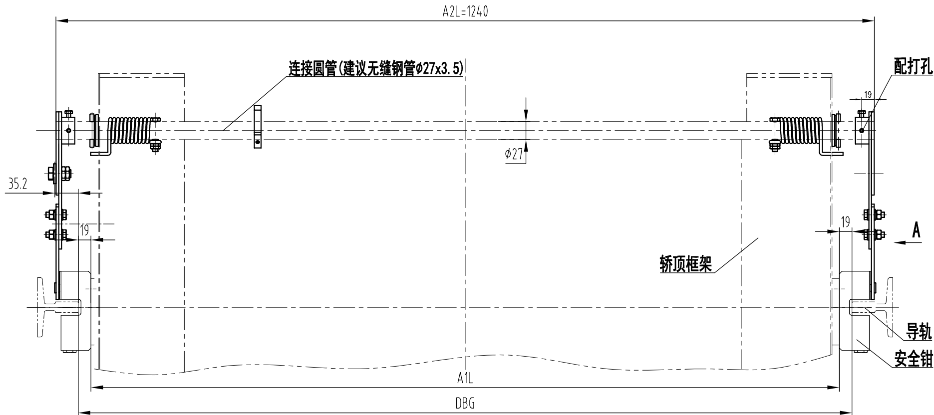
连接圆管开孔图
