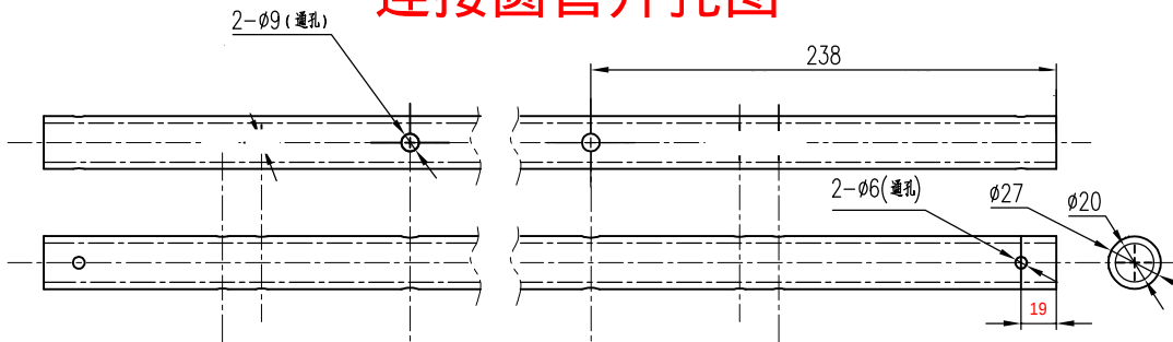
管子长1240
