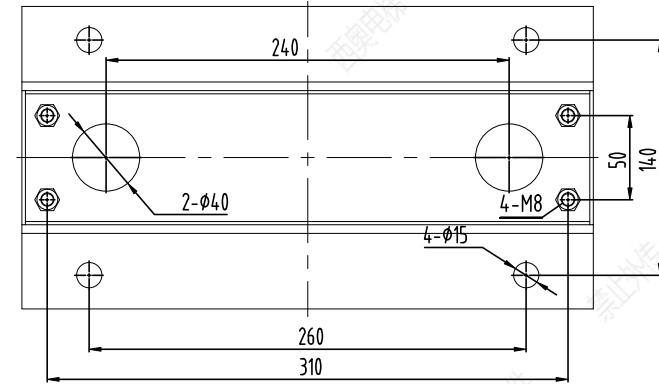
视图 A
