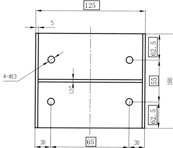
C向视图
