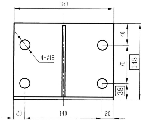
B向视图
