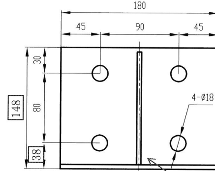
A向视图
