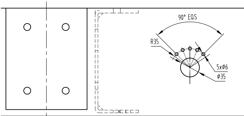
开孔尺寸
