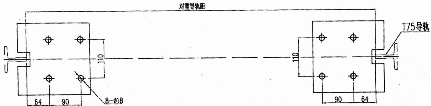
下部连接孔位示意图
