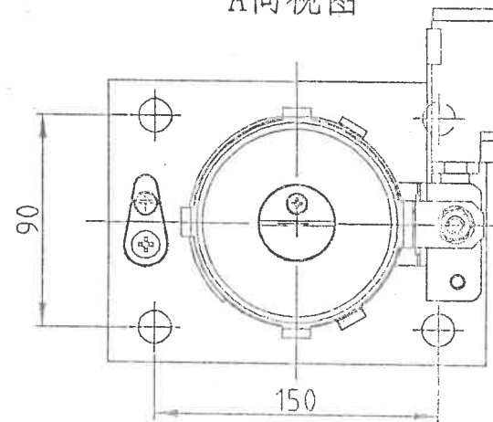
A向视图
