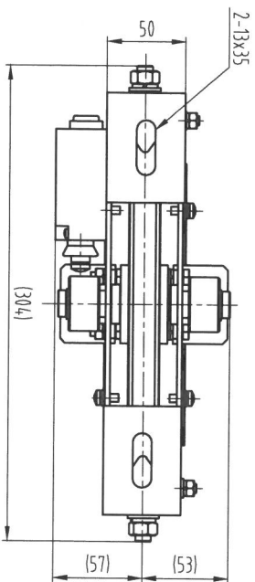
视图 A
