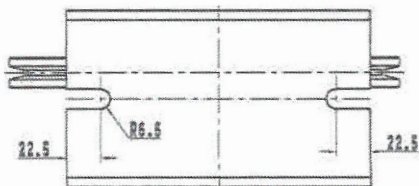
视图 A (去限速器主体配件)
