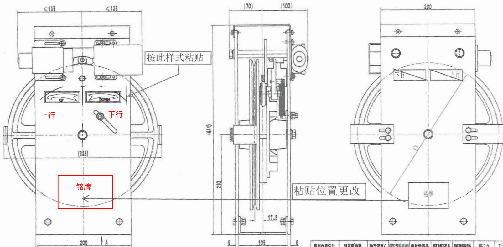
视图 A (去限速器主体配件)
