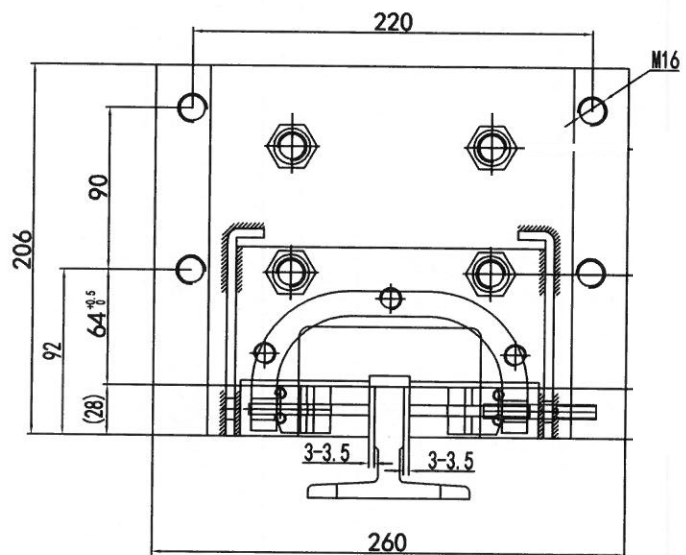
安全钳与联动装置底座连接孔
