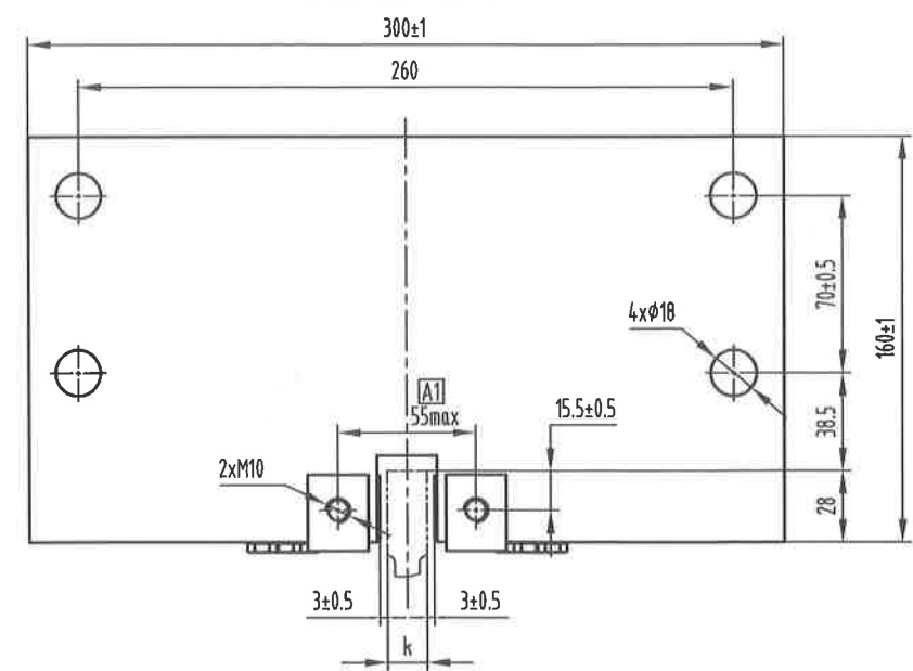
(安全钳安装面)
