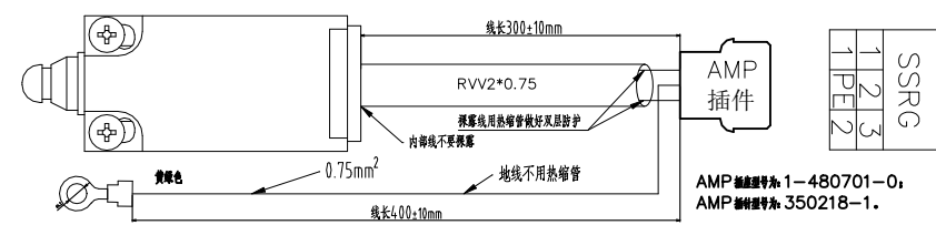
② 限速器涨紧开关接线示意图
