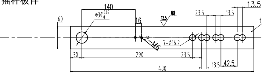
摇杆板件
