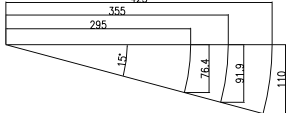
绳轮摆动尺寸示意：
