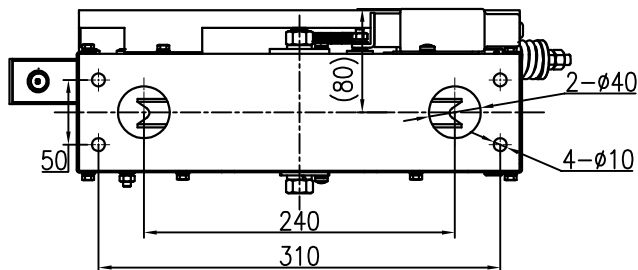
视图 A
