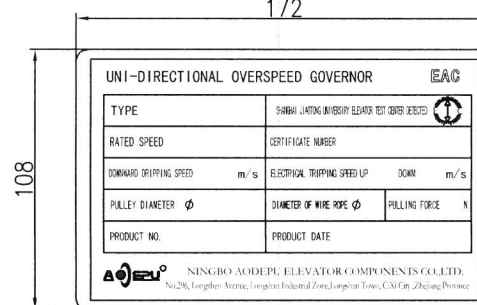
限速器英文铭牌放大图
