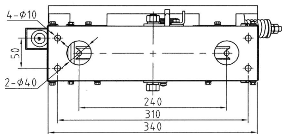
去除安装底板后视图 A
