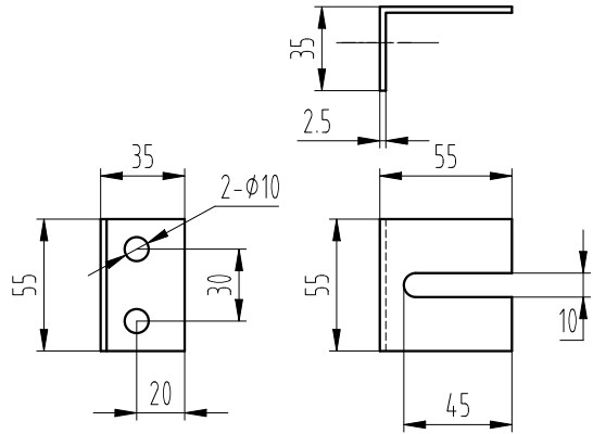
油杯支架零件示意图
