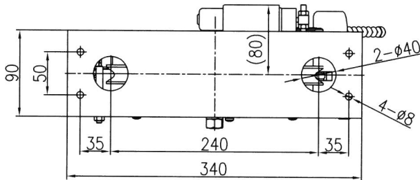
视图 A
